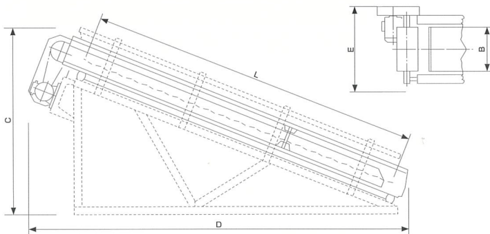
大型ダブルデッキトライソマット 2000×8400
