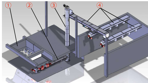
スパイラルコンベヤの応用事例 (イメージ)
