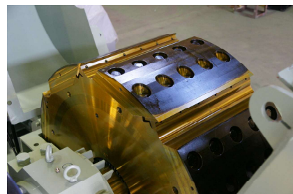
大径ロータ（φ1100mm）
