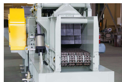
投入口（H450×W500mm）
